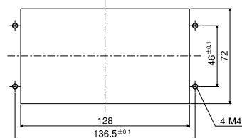
パネルカット図 For panel cut-out
