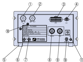
背面図 Rear view
