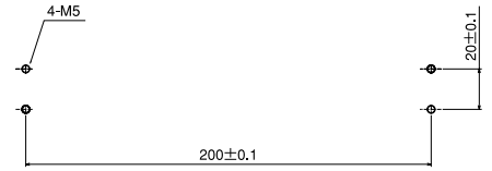
パネルカット図 For panel cut-out
